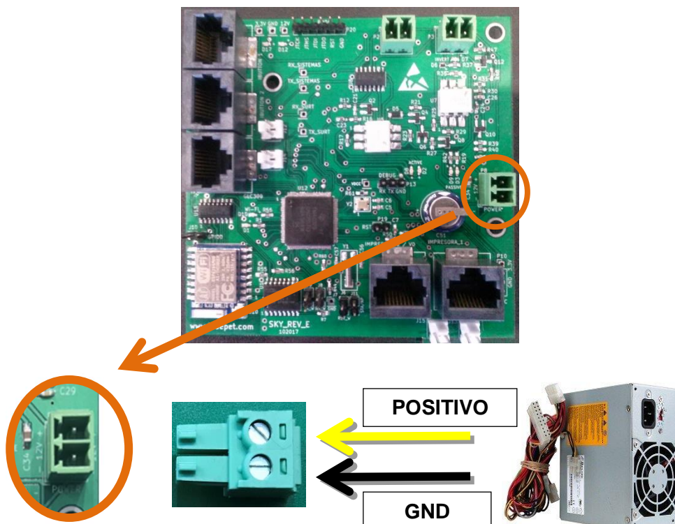
Figura 7. Conexión correcta de 12VDC.
