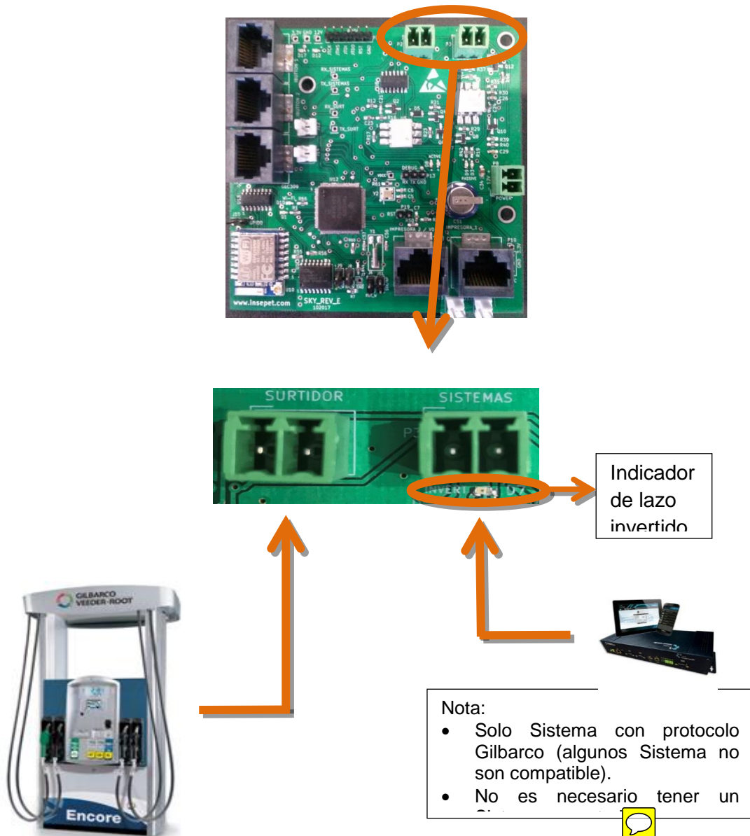
Figura 8. Instalación del Surtidor y Sistema.
